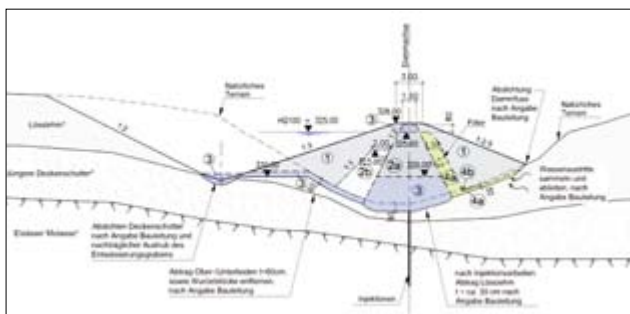
4: Typische Dammquerschnitte (Quelle: Pöyry).
