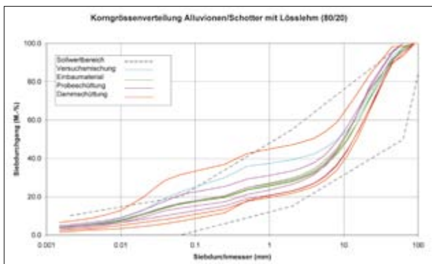
19: Siebsummenkurve der aufbereiteten Mischung aus vom Kieswerk angelieferten Alluvionen/Schotter mit natürlichem Lösslehm (80/20). Insbesondere während der Dammschüttungen traten auch hier im Bereich von 0,1 bis 10 mm Schwankungen von über 20 Masse-% auf.
