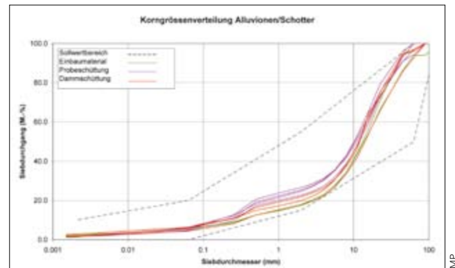
17: Der vom Kieswerk angelieferte und aufbereitete Gelbkies der Birs zeigt eine sehr homogene Zusammensetzung über alle Stadien des Dammbaus.
