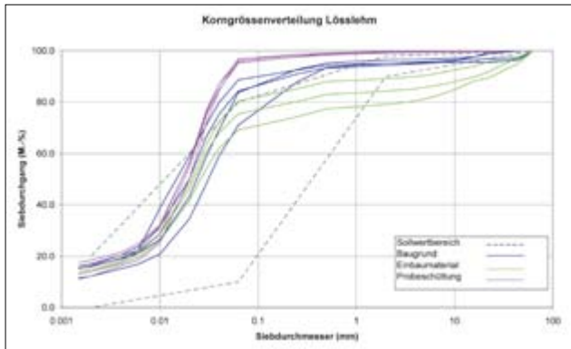
18: Siebsummenkurven Lösslehm. Das natürliche Material zeigt im Bereich von 0,1 bis 1,0 mm Schwankungen von über 20 Masse-%. Für den Einbau wurde kein reiner Lösslehm verwendet.
