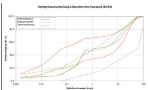
20: Durch das Mischungsverhältnis von 50/50 zwischen angeliefertem und natürlichem Material ergaben sich hier beim Einbau noch grössere Schwankungen von über 30 Masse-% im Bereich 0,1 bis 1 mm.
