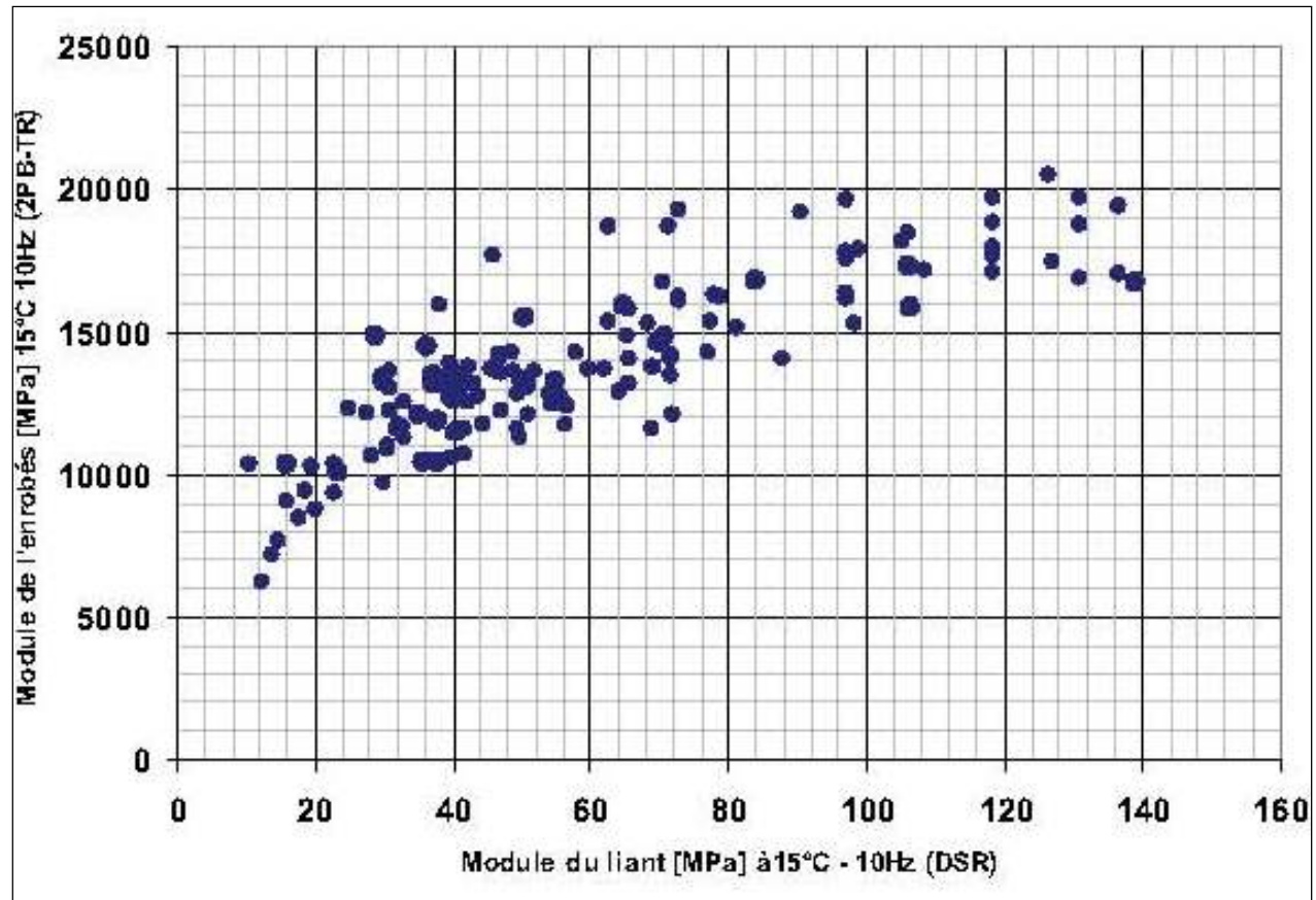
Abb. 3 Zusammenhang zwischen dem Modul des Bindemittels und dem Modul des EME-Mischgutes (J.P. Michaut; Forum Strasse 2014)
