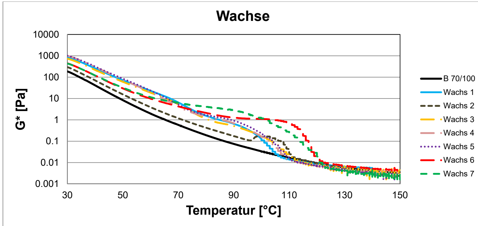
Abb 1 Gegenüberstellung verschiedener Wachse für Niedertemperatur-Asphalte (Quelle IMP)
